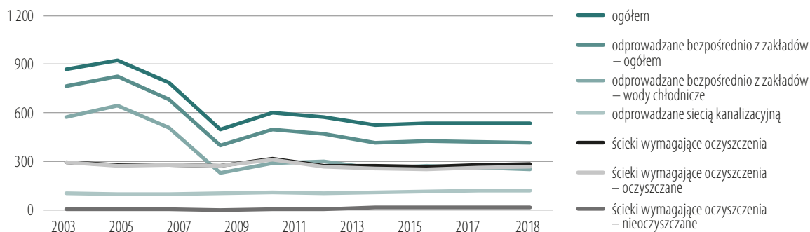
Wykres 2. Ścieki przemysłowe i komunalne odprowadzone do wód powierzchniowych lub ziemi w województwie małopolskim (hm 3 /rok)
