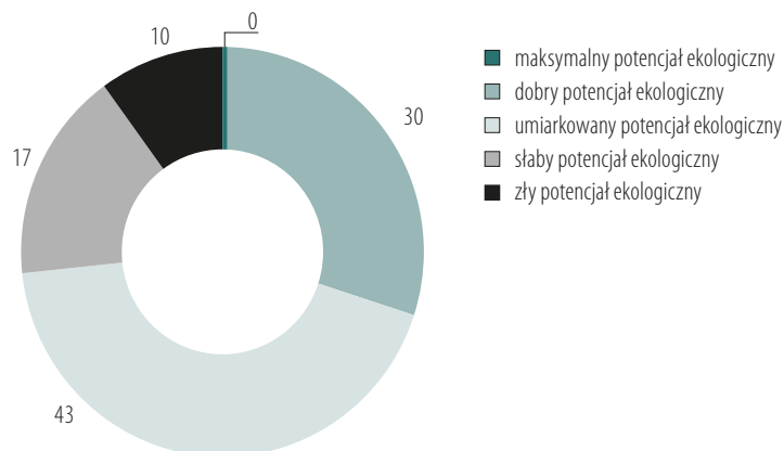
Wykres 4. Potencjał ekologiczny jcwp rzecznych monitorowanych w 2018 roku (w %)
