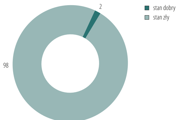
Wykres 6. Stan jcwp rzecznych monitorowanych w 2018 roku (w %)
