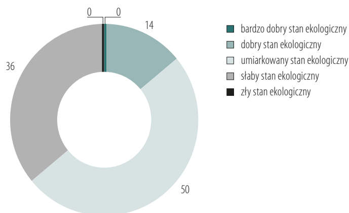
Wykres 3. Stan ekologiczny jcw rzecznych monitorowanych w 2018 roku (w %)
