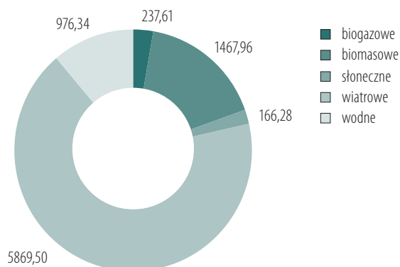
Wykres 147. Odnawialne źródła energii w Polsce w 2018 roku (moc zainstalowana [MW])
