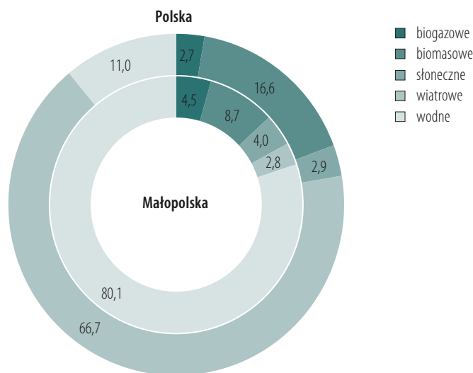
Wykres 148. Moc instalacji OZE według typu w Polsce i Małopolsce w 2018 roku (w %)
