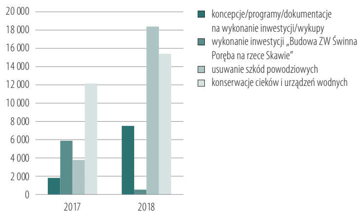
Wykres 8. Środki finansowe przeznaczane na realizację przez PGWWP RZGW w Krakowie zadań przeciwpowodziowych (w tys. zł)
