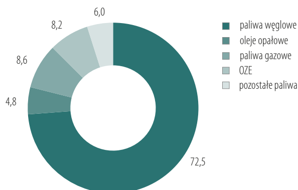
Wykres 146. Struktura paliw zużywanych w Polsce do produkcji ciepła w 2018 roku (w %)
